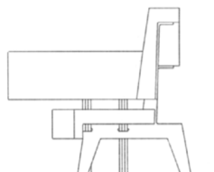
RECHTER AANZICHT
