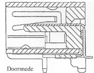
Doorsnede
