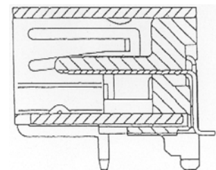
Doorsnede
