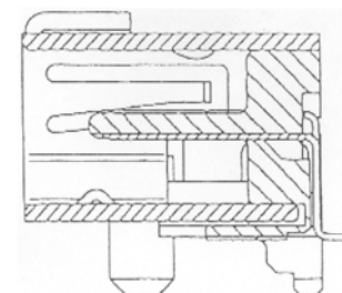
Doorsnede
