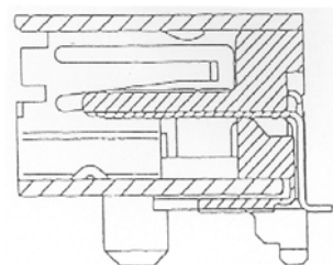
Doorsnede
