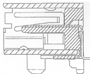
Doorsnede
