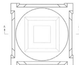
1.4 bovenaanzicht
