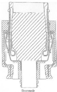
Doorsnede
