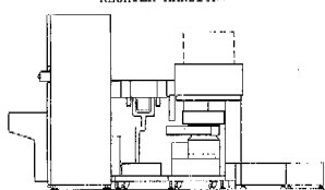
RECHTER AANZICHT
