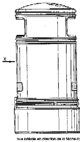
Vue frontale en direction de la lettre X cette appellation n'est pas obligatoire
