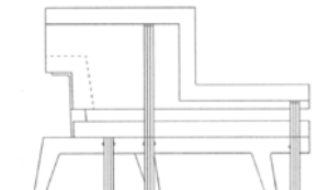
ACHTERAAZICHT
