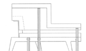
ACHTERAAZICHT
