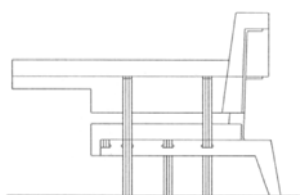
RECHTER ZIJAAZICHT
