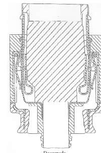
Doorsnede
