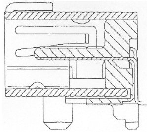
Doorsnede
