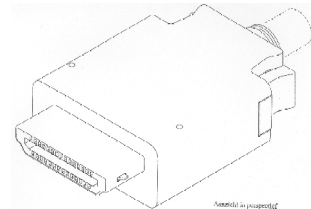
Aanzicht in perspectief
