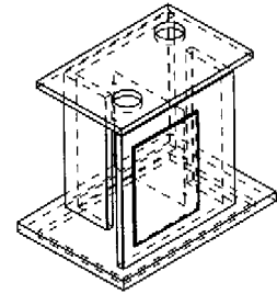
ISOMETRIE
