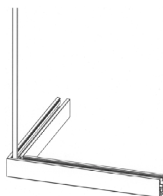
Perspectief detail
