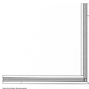
Horizontale doorsnede
