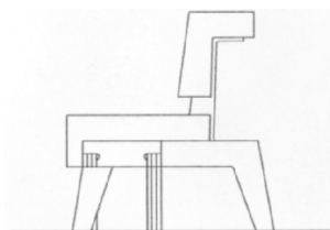
RECHTER ZIJAAANZICHT
