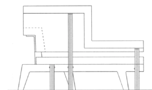
ACHTERAANZICHT
