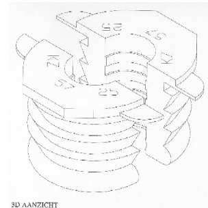
3D AANZICHT
