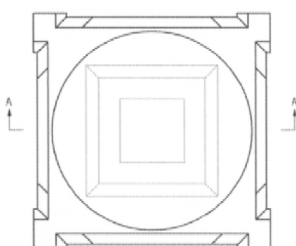
1.4 bovenaanzicht
